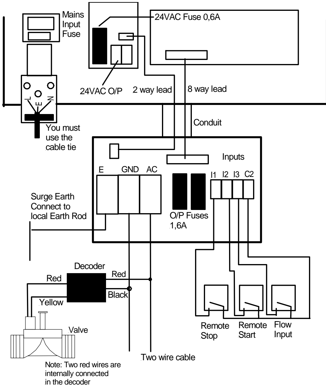
Fig 1 Output Wiring
